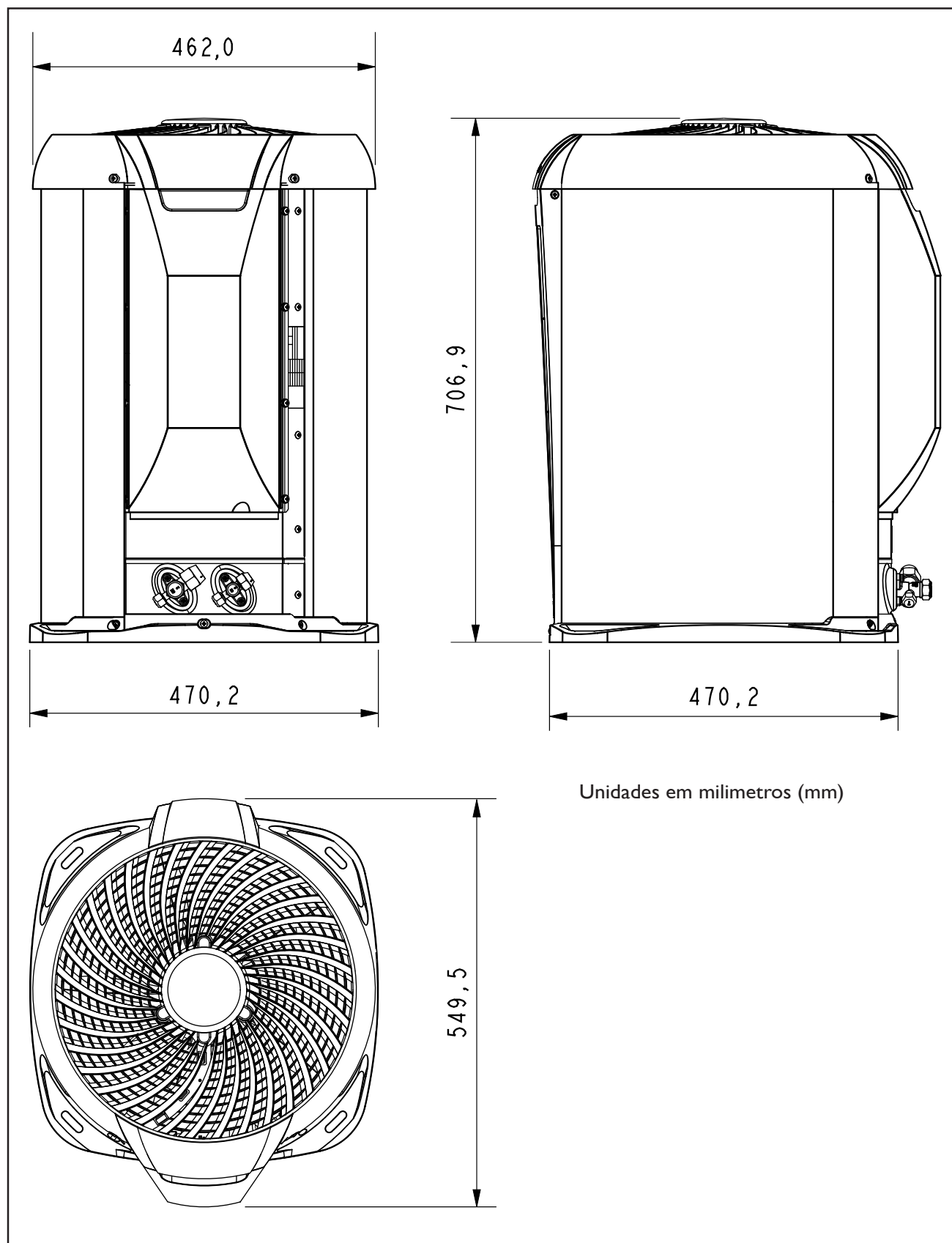
FIG. 12 - DIMENSIONAL UNIDADE CONDENSADORA 38TF_24
