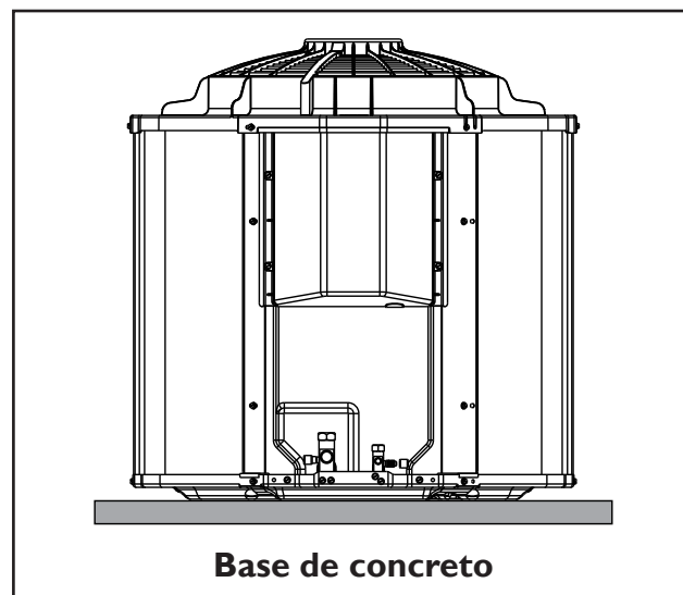
FIG. 4 - CALÇOS RECOMENDADOS PARA UNIDADES CONDENSADORAS
