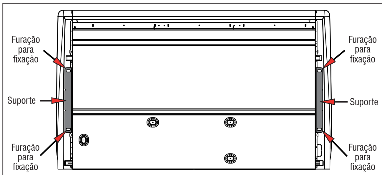
FIG. 21 - SUPORTES E FURAÇÃO PARA FIXAÇÃO
