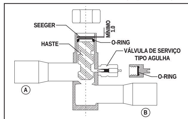
FIG. 32 - VÁLVULA DE SERVIÇO ABERTA
