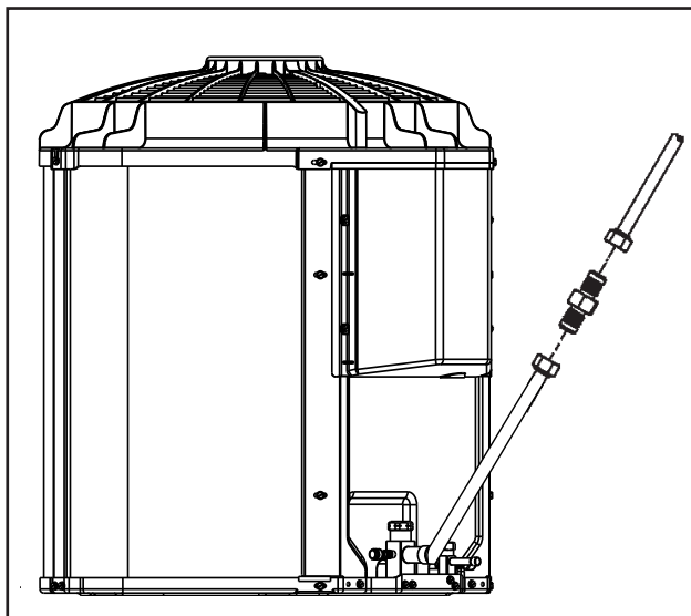
FIG. 45 - INSTALAÇÃO DO KIT SISTEMA DE EXPANSÃO
