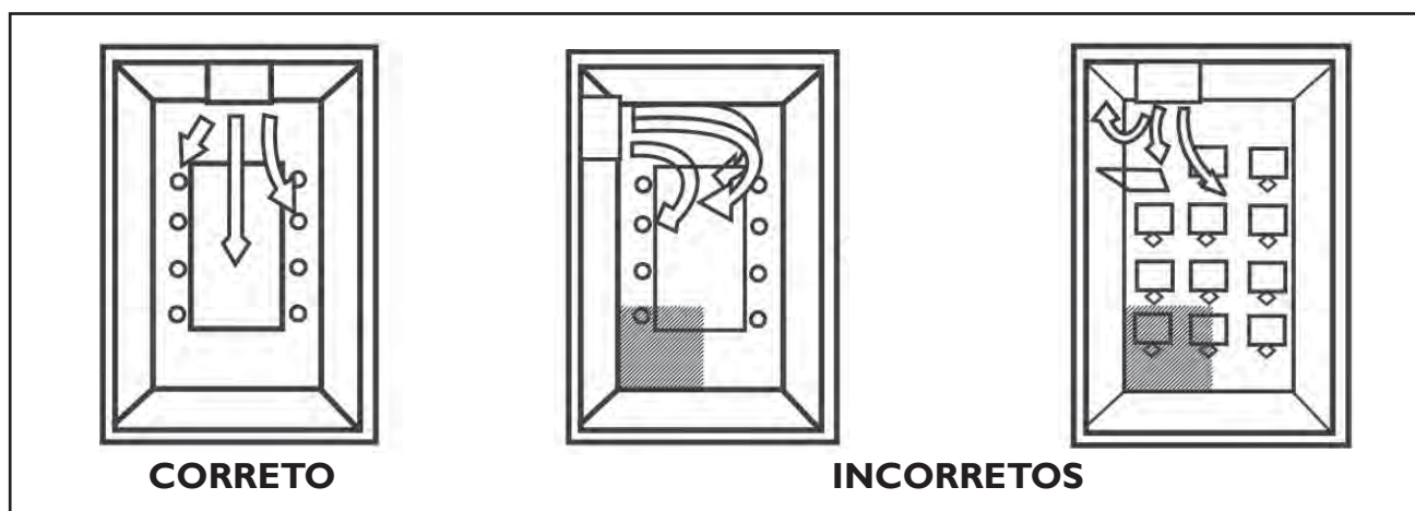
FIG. 20 - POSIÇÃO DA EVAPORADORA NO AMBIENTE
