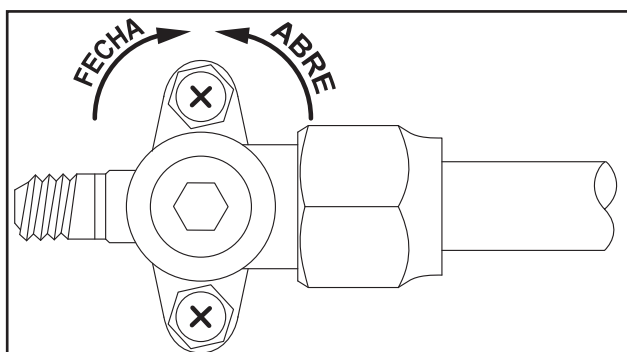
FIG. 30 - VÁLV. SERVIÇO SEM A PORCA DE PROTEÇÃO
